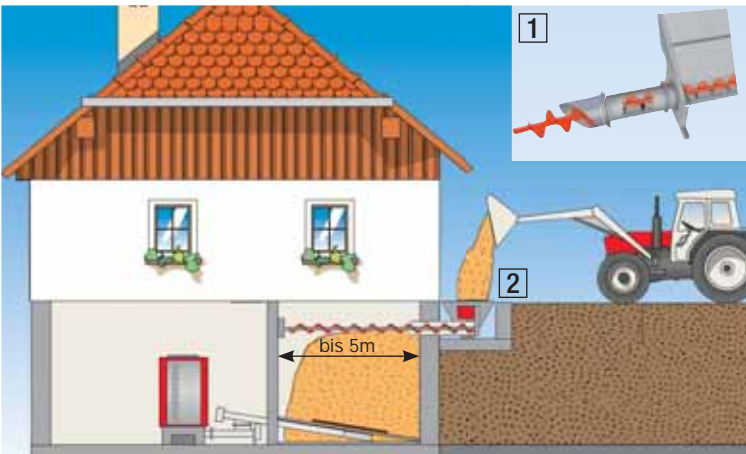
Für Kellerräume mit versenktem Trog und waagrechter Befüllschnecke, fix mit Lager montiert
